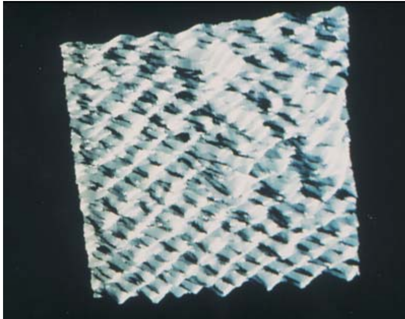
1993D00521 - © CNRS Photothèque - La microscopie tunnel permet de mettre en évidence la structure superficielle des alliages à l'échelle atomique.
