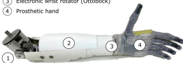
Prototype de prothèse de bras utilisé pour les essais, composé d'un coude motorisé (1), d'un rotateur motorisé de poignet (3) et d'une main polydigitale Robolimb de Touch Bionics (4).
