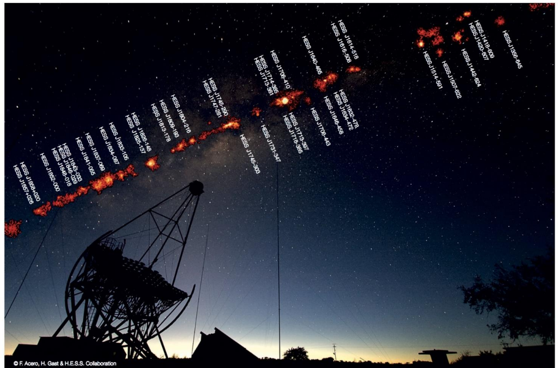
Montage représentant les sources de rayons gamma de très haute énergie de la Voie Lactée au dessus des télescopes H.E.S.S. en Namibie. (Photographie de la Voie Lactée au dessus des télescopes H.E.S.S. en Namibie: © F. Acero, / Cartographie des sources Gamma: © H.E.S.S. Collaboration)
