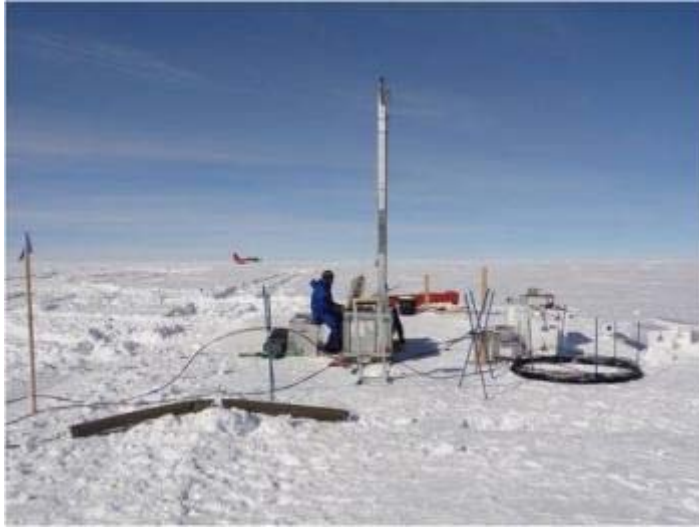
Forage-Point-Barnola : photo prise le 18 janvier, jour où Manu et Martin étaient récupérés avec le Twin que l'on voit au fond (posé sur une piste faite pour l'occasion avec le Kassbohrer). On voit le carottier 200 m en position de forage. Au premier plan le manchon gonflable, avec les tubes Dekabon pour les prélèvements d'air enroulés à droite. (Photo J. Chappellaz/LGGE)
