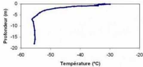
Profil de température dans la neige à S2 28 décembre 2011
