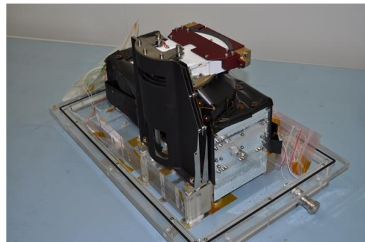
Modèle structurel et thermique de l'instrument PAS. Il est pleinement représentatif de l'encombrement, de la masse et des propriétés thermiques de l'instrument. Ce modèle a été testé sous un flux solaire représentatif de 10 constantes solaires. Crédit : IRAP
