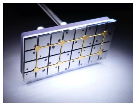
Module XRDPIX constitué de 32 détecteurs de tellure de cadmium de 4mm de côté. Le plan de détection de l'instrument ECLAIRs sera constitué de 200 modules de ce type.
