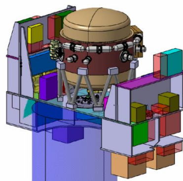
Schéma de l'instrument X-IFU Crédit : I. Maussang et T. Lam-Trong
