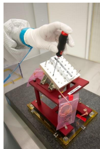
Modèle de vol de l'instrument IDEE en cours de qualification à l'IRAP. © Sébastien CHASTANET / OMP / IRAP / CNRS Photothèque
